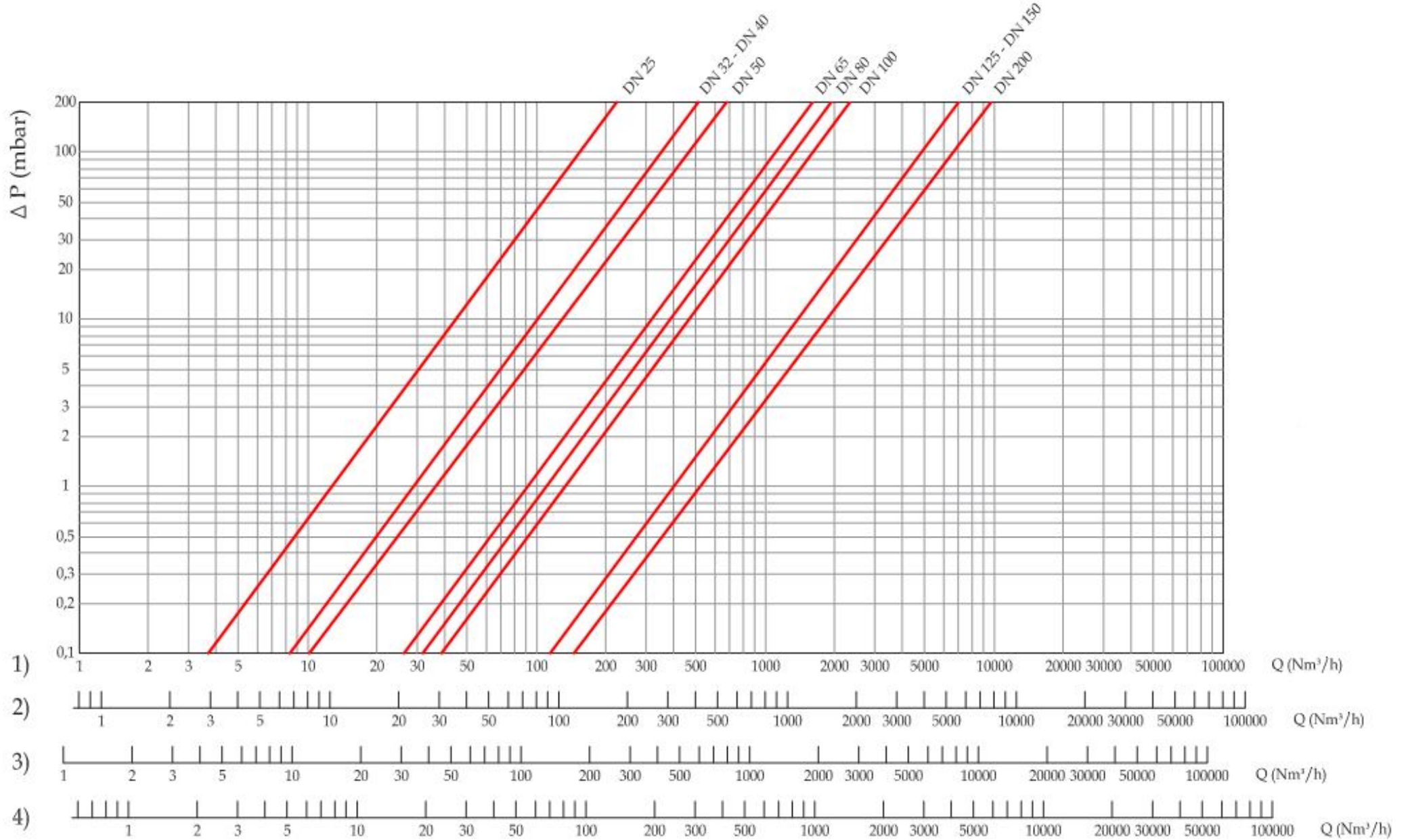
SOLENOİD VANA KAPASİTE TABLOSU (1.METAN, 2. HAVA, 3. DOĞAL GAZ, 4. LPG)
